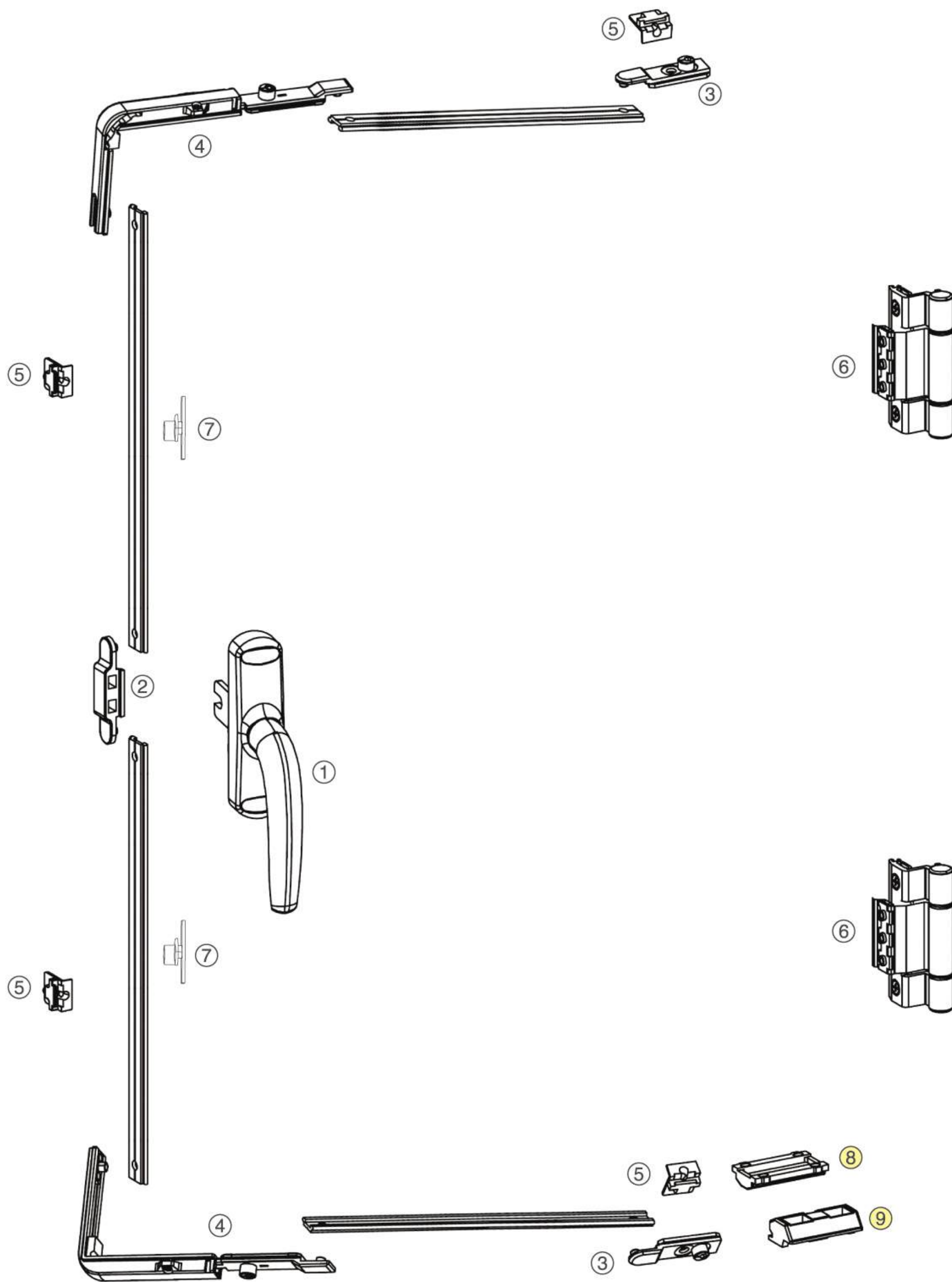
欧槽内开四点锁五金件配置表
