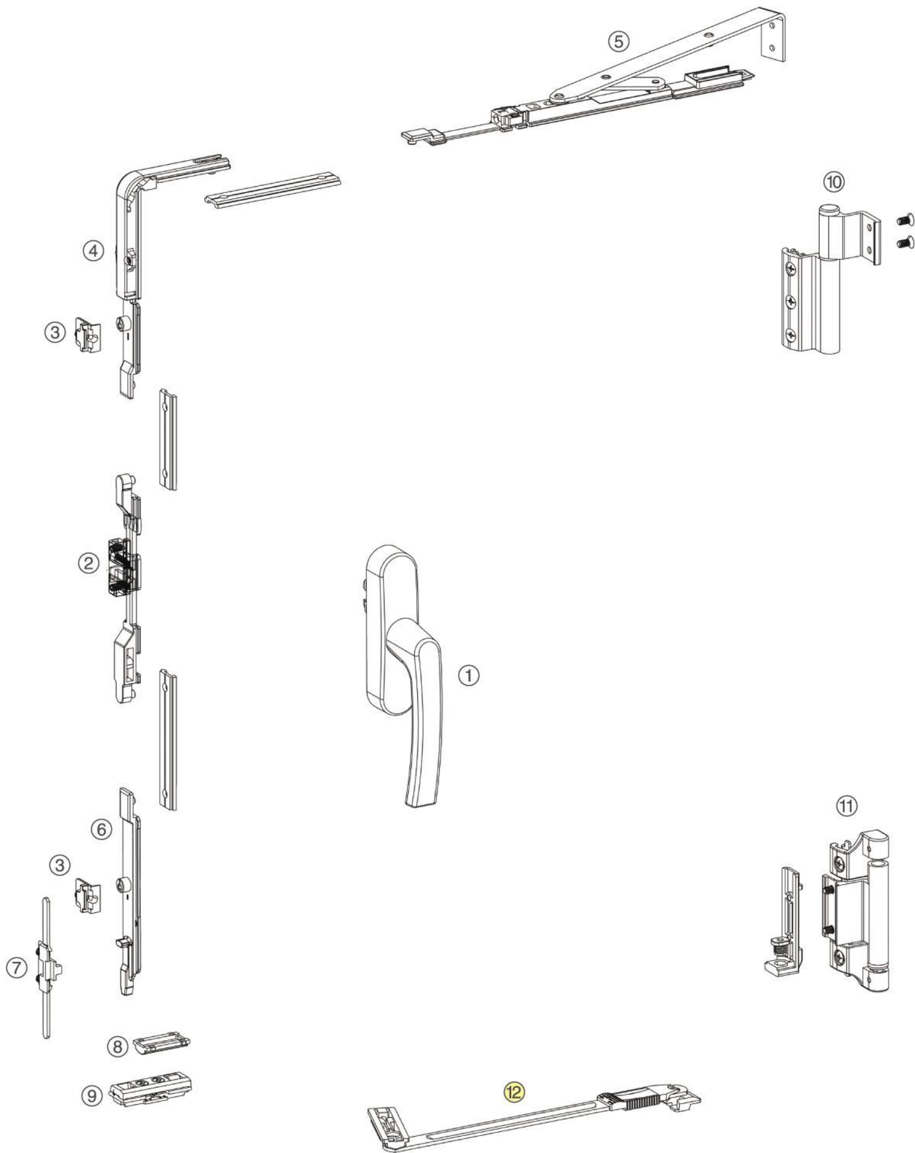
欧槽内开内倒五金件配置表
